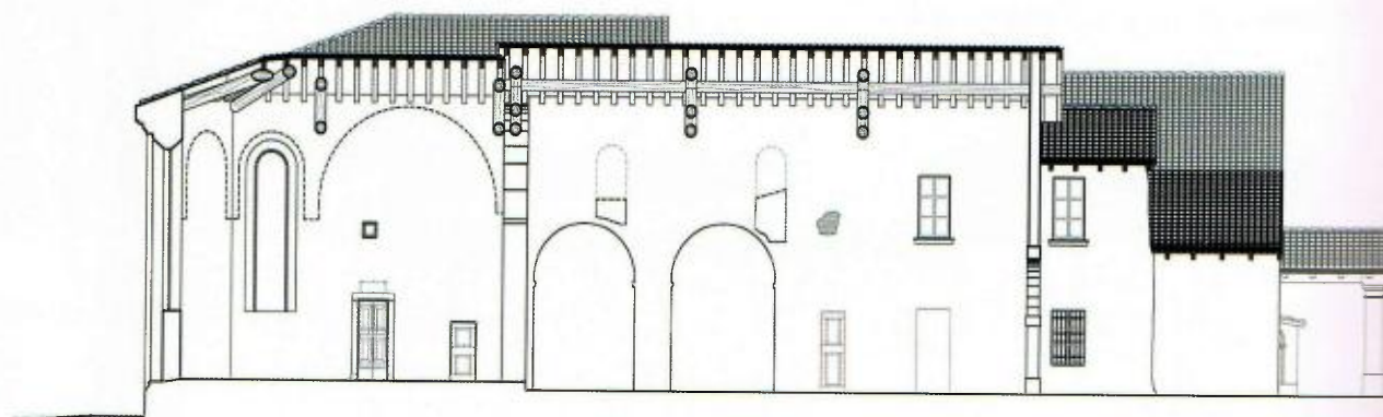
Sezione est-ovest chiesa
