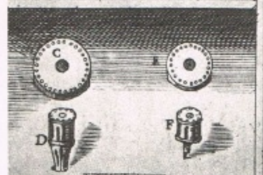
Il mulino da seta nella sua prima rappresentazione storica. La tavola mostra la struttura rotante interna della macchina. (Da V. Zonca, op. cit.).
